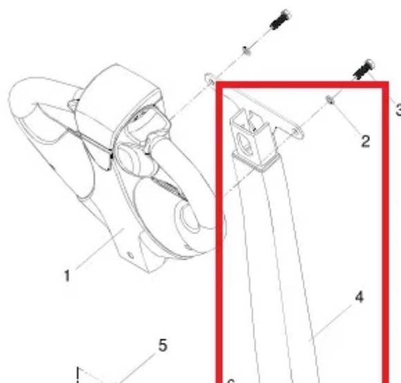
图 4 操纵转向系统 Fig.4 Tiller handle assy
